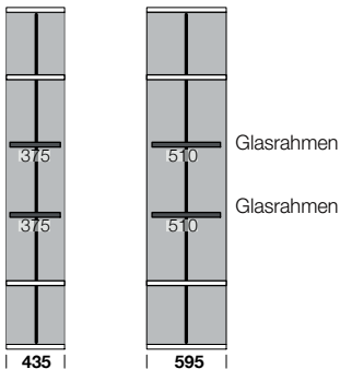
BÜNDIGE HOLZEINLEGEBÖDEN SEITENWAND ZURÜCKSTEHENDE RAHMENEINLEGEBÖDEN 2-SEITIG Querschnitt
