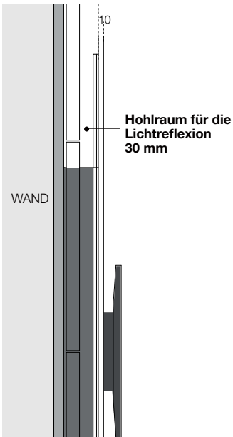
ABSCHNITT WANDPANEEL ST. 25
