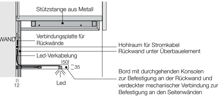
Rückwandabschnitt mit Griff B 1325-1475-1775-1975-2075-2175-2375
