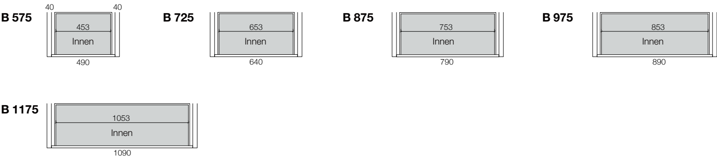
GRUNDRISS
