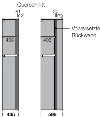
ZURÜCKSTEHENDE HOLZ- ODER RAHMENEINLEGEBÖDEN
