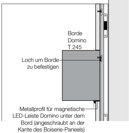
BORDE DOMINO
