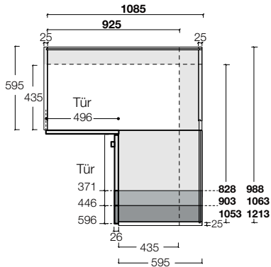
Eckanbaumodul 1085-925
