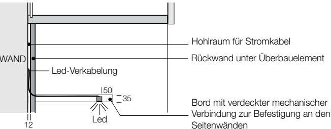
Rückwandabschnitt mit Griff B 425-475-575-725-875-975-1175
