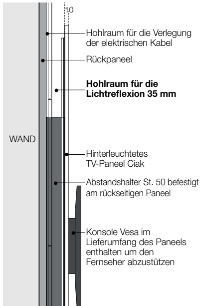
ABSCHNITT WANDPANEEL ST. 10/12
