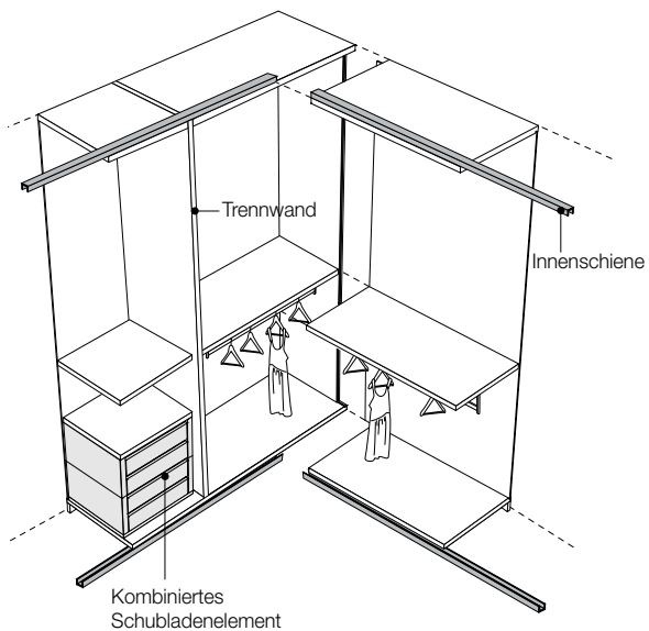
MIT INNENSCHUBKÄSTEN IM FACH, DAS DURCH DIE INNENAUFTEILUNG ENTSTANDEN IST (FÜR ECKEN MIT TÜREN IN B 1020 UND B 1220)
