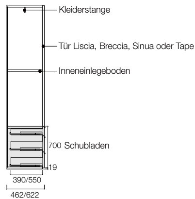
Modul 3 Schubladen
