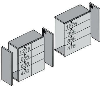
KOMPLETTER HÄNGESCHRANK
