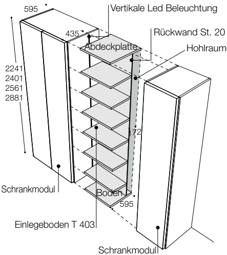
FRONTSEITIGES BÜCHERREGAL
