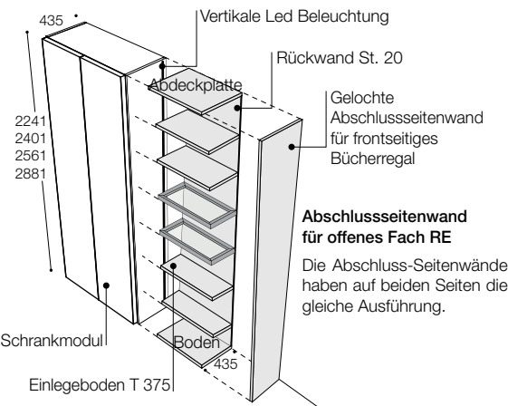
FRONTSEITIGES ZWEISEITIGES DURCHGEHENDES ABSCHLIESSENDES BÜCHERREGAL
