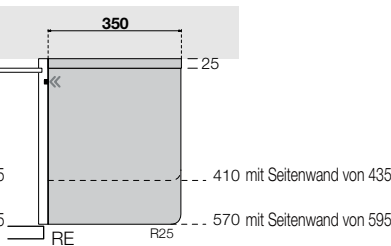
MODULE L 350
