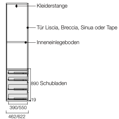
Modul 4 Schubladen
