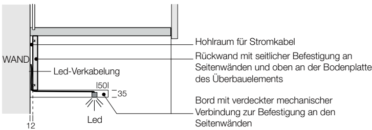
Querschnitt Bord mit kleiner Rückwand B 425-475-575-725-875-975-1175
