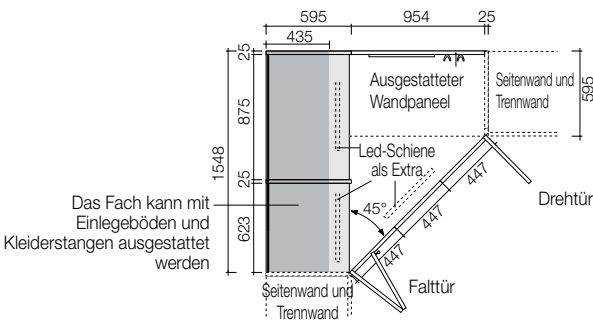
GRUNDRISS UMKLEIDERAUM "C" RE
