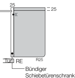
NEBENEINANDERSTELLUNG MIT MODUL MIT SCHIEBETÜR (Innentür)
