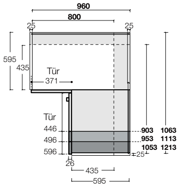
Eckanbaumodul 960-800
