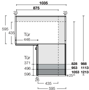
Eckanbaumodul 1035-875
