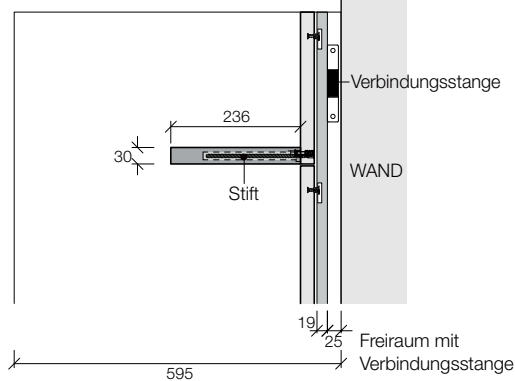
BORD ST 30 MIT GERADER KANTE
