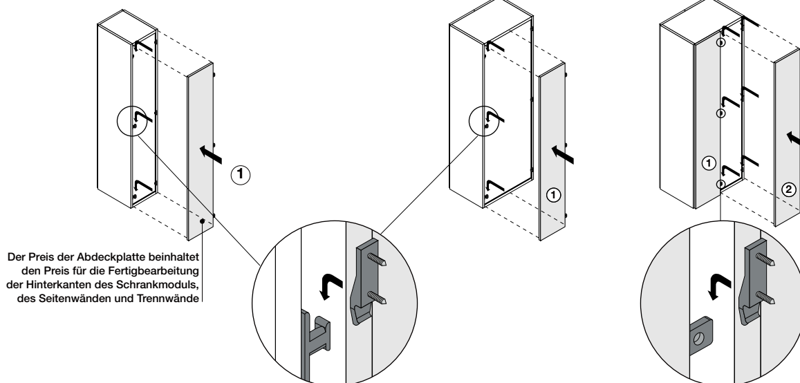
MODUL 1 TÜREN
