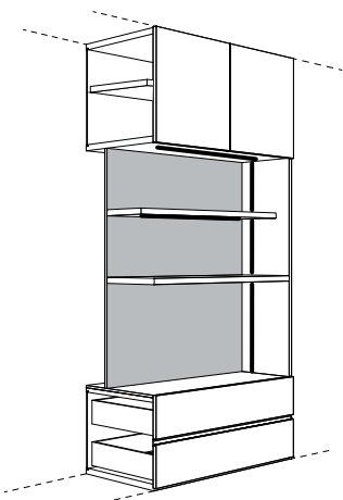
ELEMENT TECA T 622 mit zurückversetzter Zwischenrückwand
