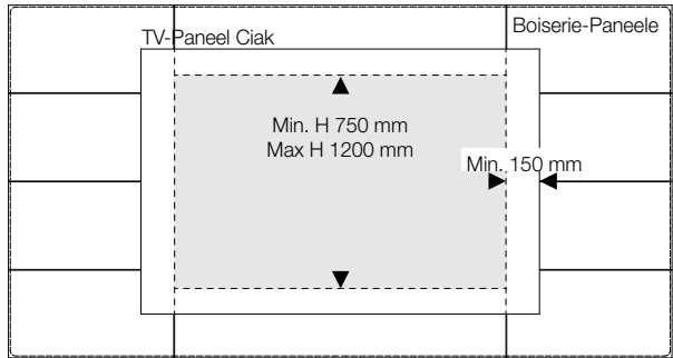
VORDERANSICHT
