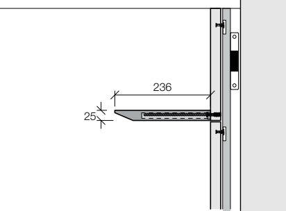
BORD ST 25 MIT 45°-KANTE
