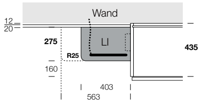
GRUNDRISS T 275/350
