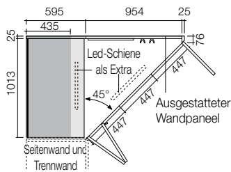
GRUNDRISS UMKLEIDERAUM "A" RE
