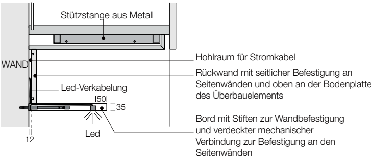
Querschnitt Bord mit kleiner Rückwand B 1325-1475-1775-1975-2075-2175-2375
