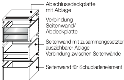
Beispiel 1 montiert
