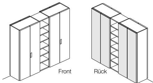
Doppelseitig DURCHGEHEND mit offenes Modul IN DER MITTE
