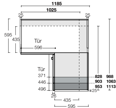
Eckanbaumodul 1185-1025
