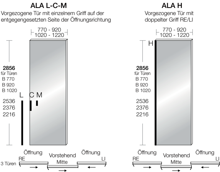
Abschnitt Tür ALA LISCIA
