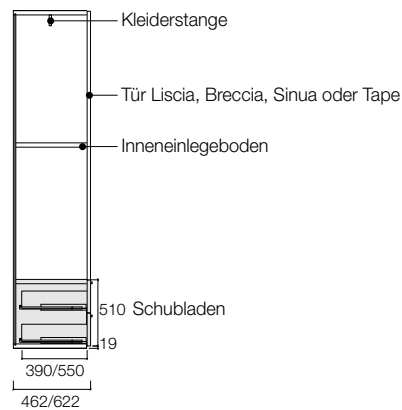
Modul 2 Schubladen
