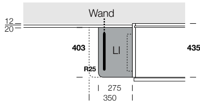
GRUNDRISS T 403/563
