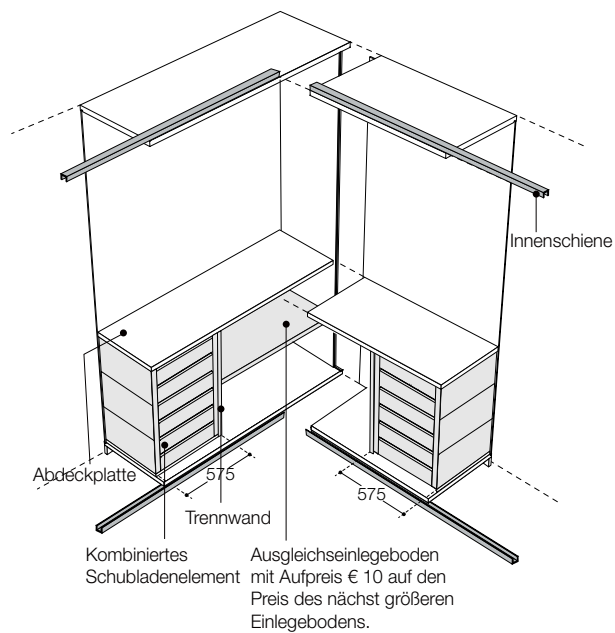
MIT ÜBEREINANDERSTEHENDEN INNENSCHUBKÄSTEN UND TRENNWAND
