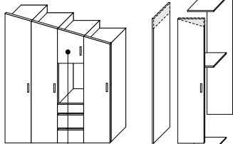
Mindesthöhe der Tür H 316 mit Abschlusswinkel
