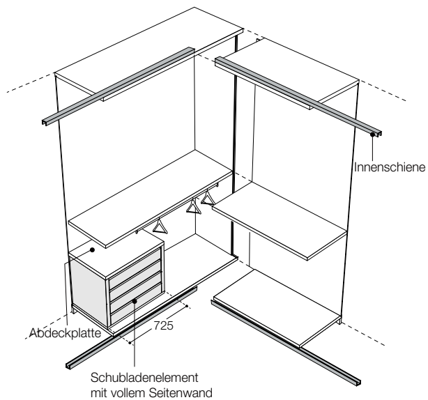
MIT SELBSTTRAGENDEN INNENSCHUBLADENELEMENT
