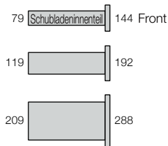
SCHUBLADENHÖHE
