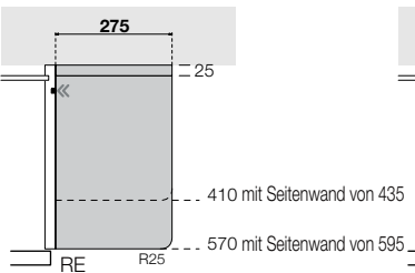
MODULE L 275
