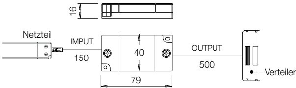
EMPFÄNGER für Fernbedienungen DIMMER
