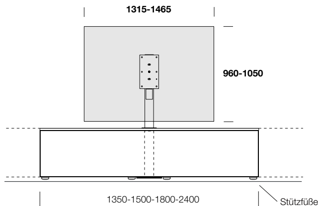
Bodenstehender Unterschrank mit Stützfüßen
