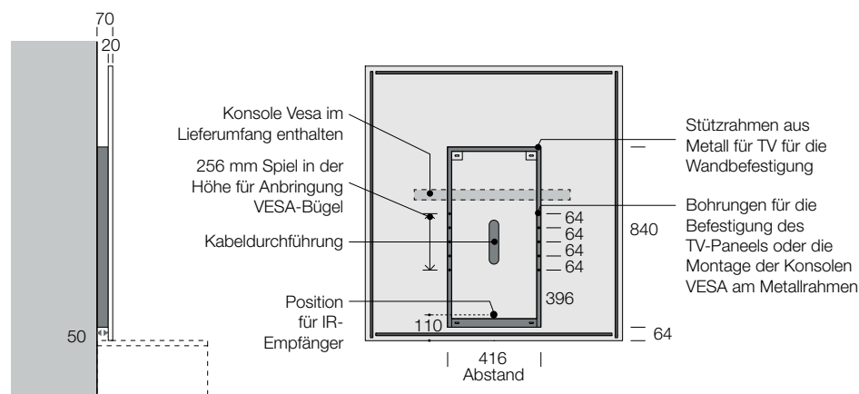
PANEEL ST 20 MIT RAHMEN für Breiten 1350-1500
