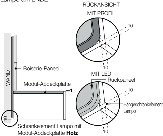
Schränkelement Lampo am ENDE
