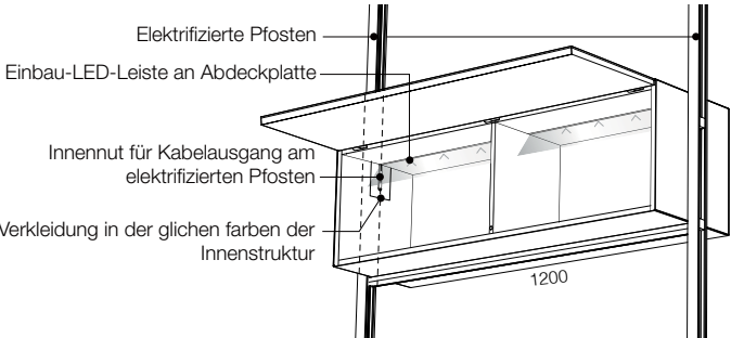
INTERNE, IN DER DECKPLATTE DES ELEMENTS LAMPO EINGELASSENE LED-LEUCHTE MIT TRENNWAND
