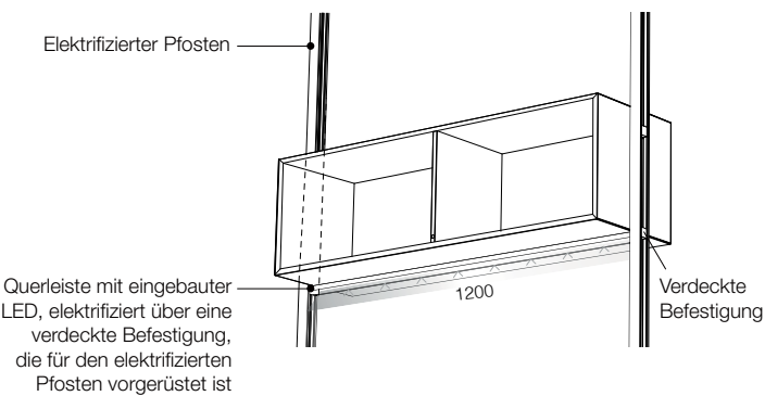
EXTERNE, IN DER QUERSTREBE EINGELASSENE LED-LEUCHTE MIT EINZELNER KABELAUSGANG
