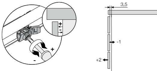
Tiefeneinstellung für Push-Pull
