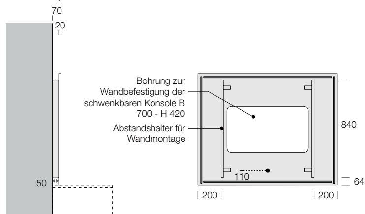
PANEEL ST 20 MIT ABSTANDLEISTEN - Mit Bohrung für schwenkbare TV-Wandhalterung - Abschlusspaneel
