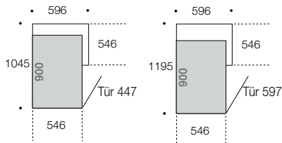
AUSSENMASSE ECKUNTERSCHRANK T 546 mm LINKS
