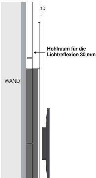
ABSCHNITT BOISERIE ST. 25
