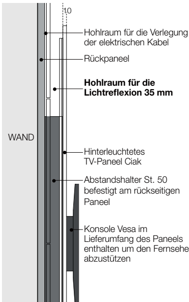
ABSCHNITT BOISERIE ST. 10/12
