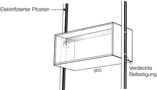
INTERNE, IN DER DECKPLATTE DES ELEMENTS LAMPO EINGELASSENE LED-LEUCHTE
