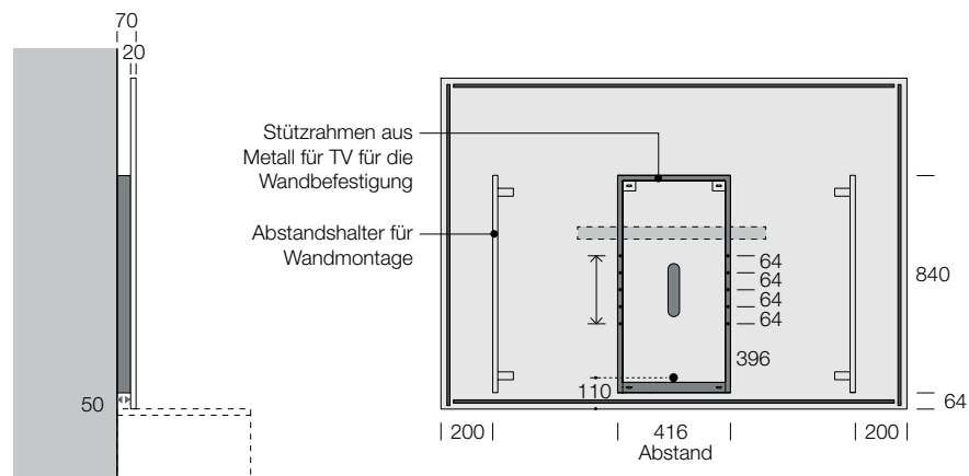
PANEEL ST 20 MIT RAHMEN UND ABSTANDLEISTEN für Breiten 1800-2100-2400
