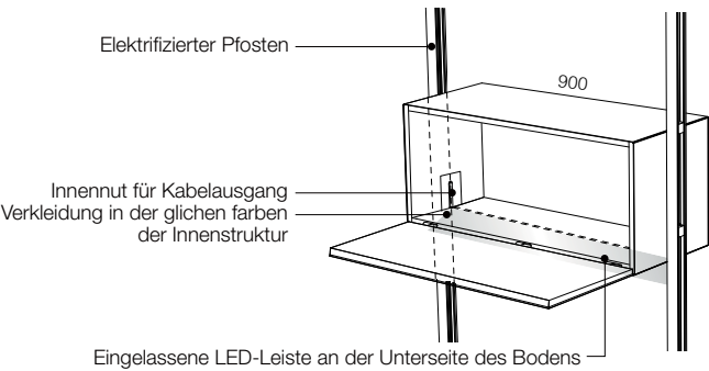
EXTERNE, AUF DER UNTERER SEITE DER BODEN VON ELEMENTE LAMPO EINGELASSENE LED-LEUCHTE
