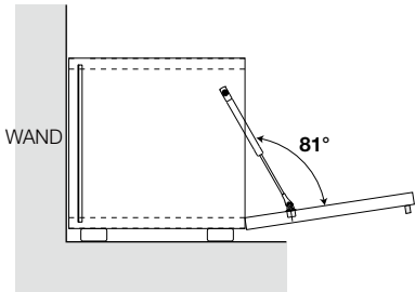
Klapptür nach unten für Bodenstehende Elemente
