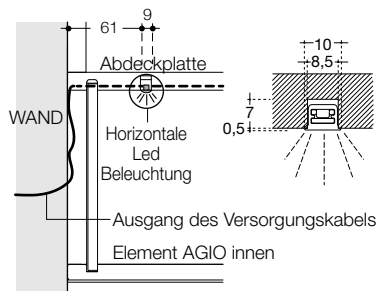
ABSCHNITT HORIZONTALE LED-LEISTE
