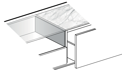
Seitliche Tragwand neben Element mit modularer Abdeckplatte aus Keramik
