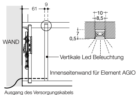
ABSCHNITT VERTIKALE LED-LEISTE
