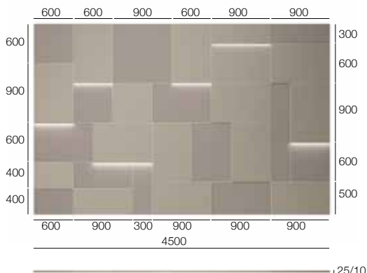
B 4500 x 2900 x ST 10/25
