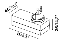
Ingombro del trasformatore (plug escluso). LED driver dimensions (plug excluded)
